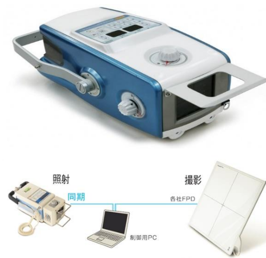
車載のポータブルX線装置一式
