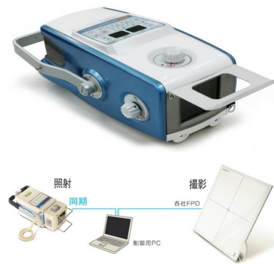
車載のポータブルX線装置一式
