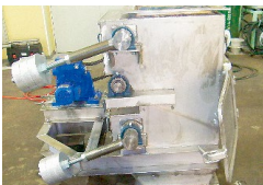
フラップダンパー
